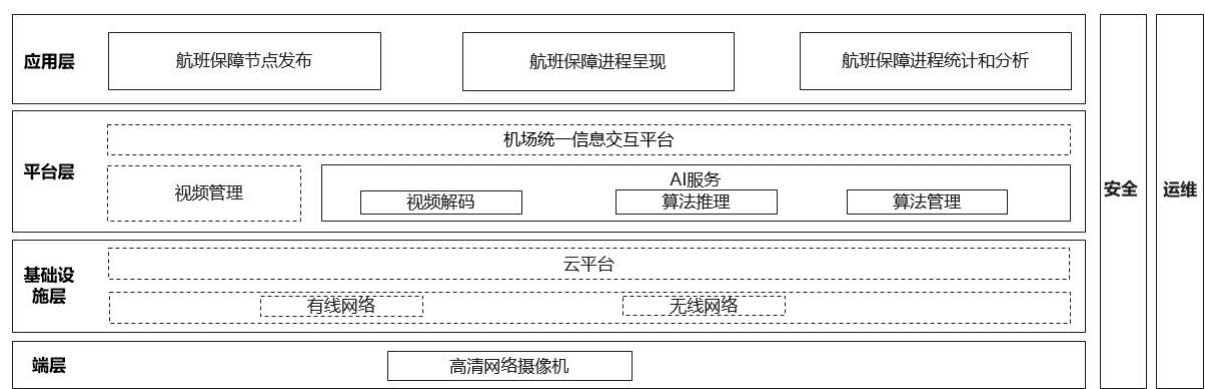
图 1 基于视频分析的航班保障节点采集系统技术架构
