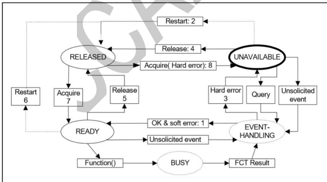
图 4 设备组件状态图（航司应用视图）
