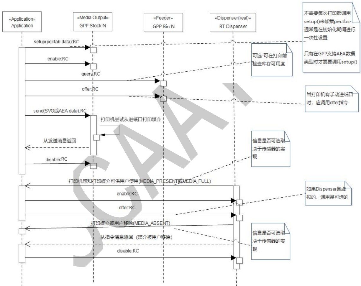
图 13 GPP 打印机的典型序列图
